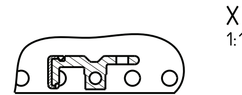
Ausführung 1: Hintere Verbindungsschienen für Busplattenmontage
