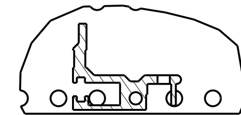
Ausführung 2: Hintere Verbindungsschienen für Einzelsteckverbinder
